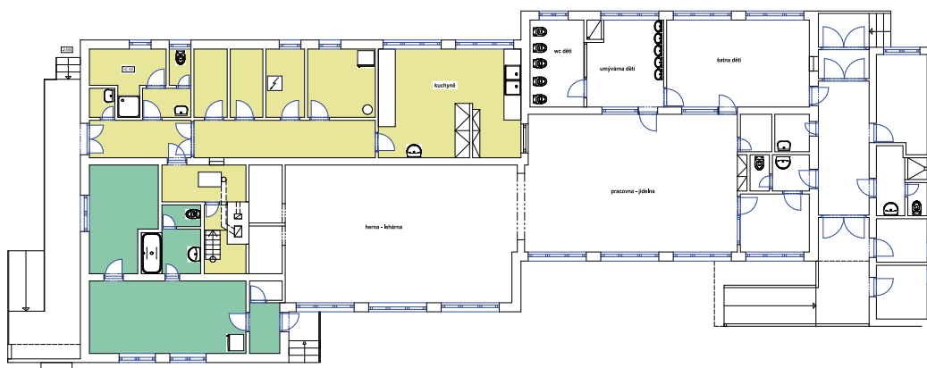
PŮDORYS 1.NP_ NÁVRH ÚPRAV
